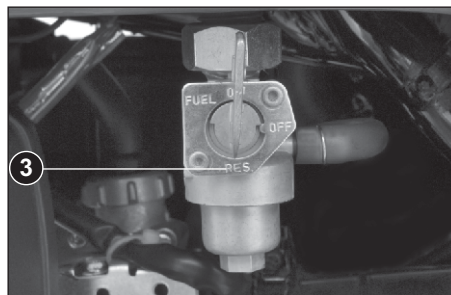
(3) Posicion "RES"
