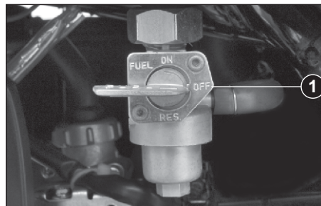
(1) Posición "OFF"
